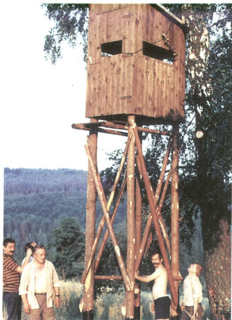
Budowa ambony
