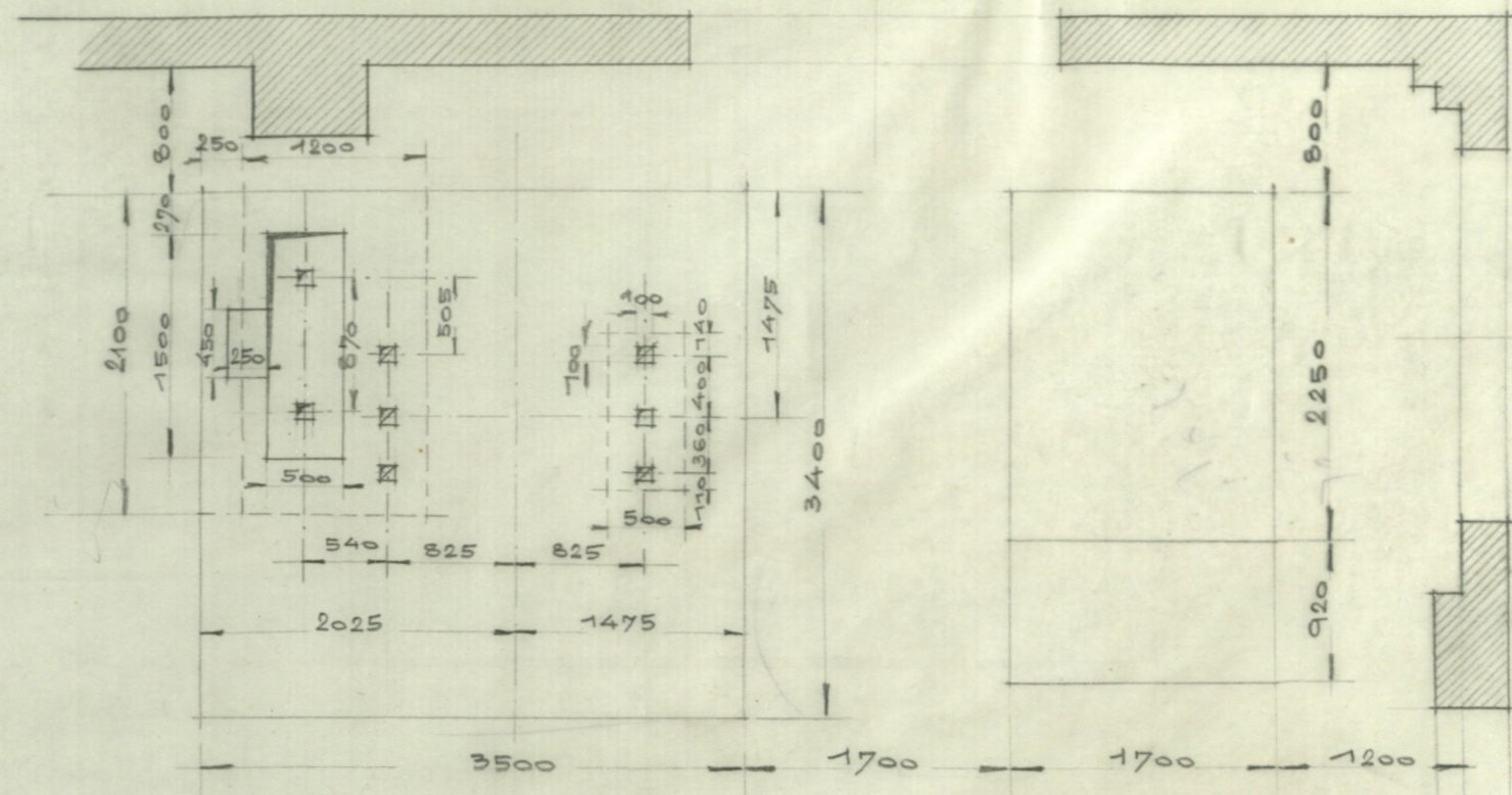
Montage-halle.
