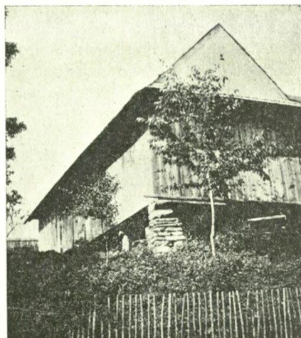
Fundament słupowy, podpierający jeden róg.
